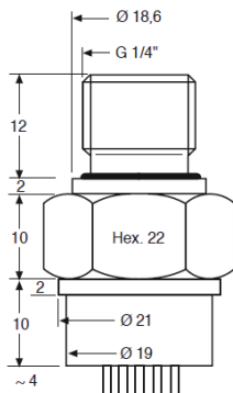
6 S: 0,3...200 бар
