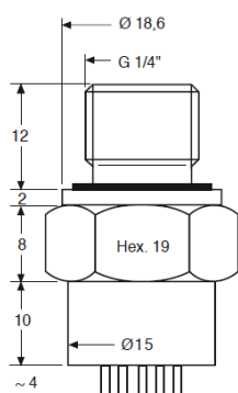
6 S / 6 М: 5...200 бар (Компактная версия)
